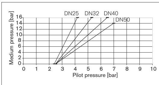
Actuator Ø 90
